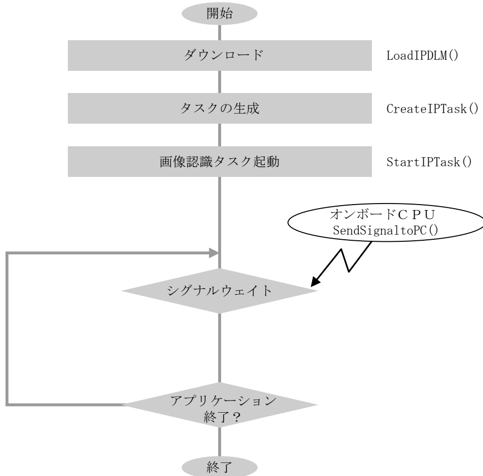
図6-3-3 画像認識タスクモジュール制御フロー
