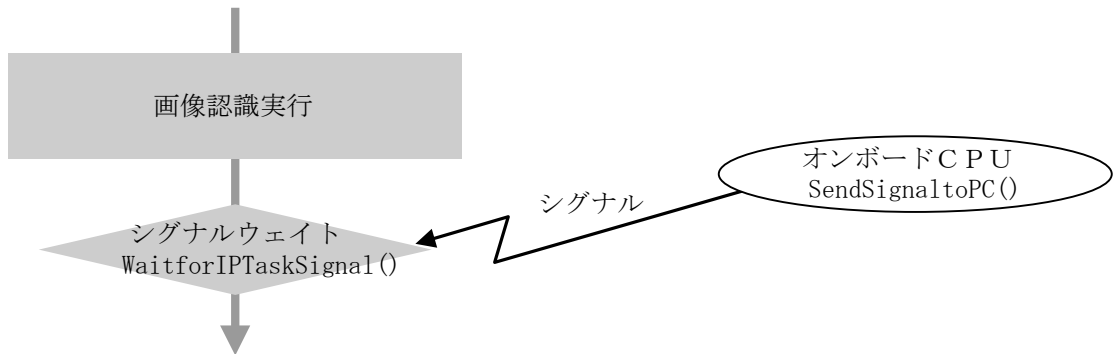
図6-3-2 PCとの同期
