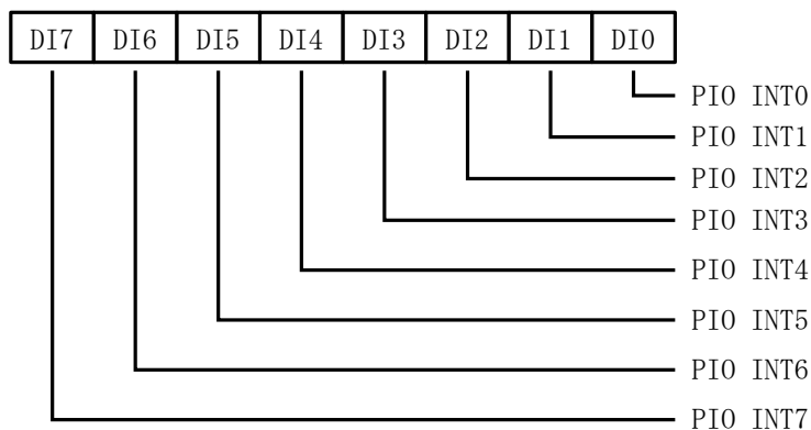
図6-4-2 PIO入力ポートの割り当て
