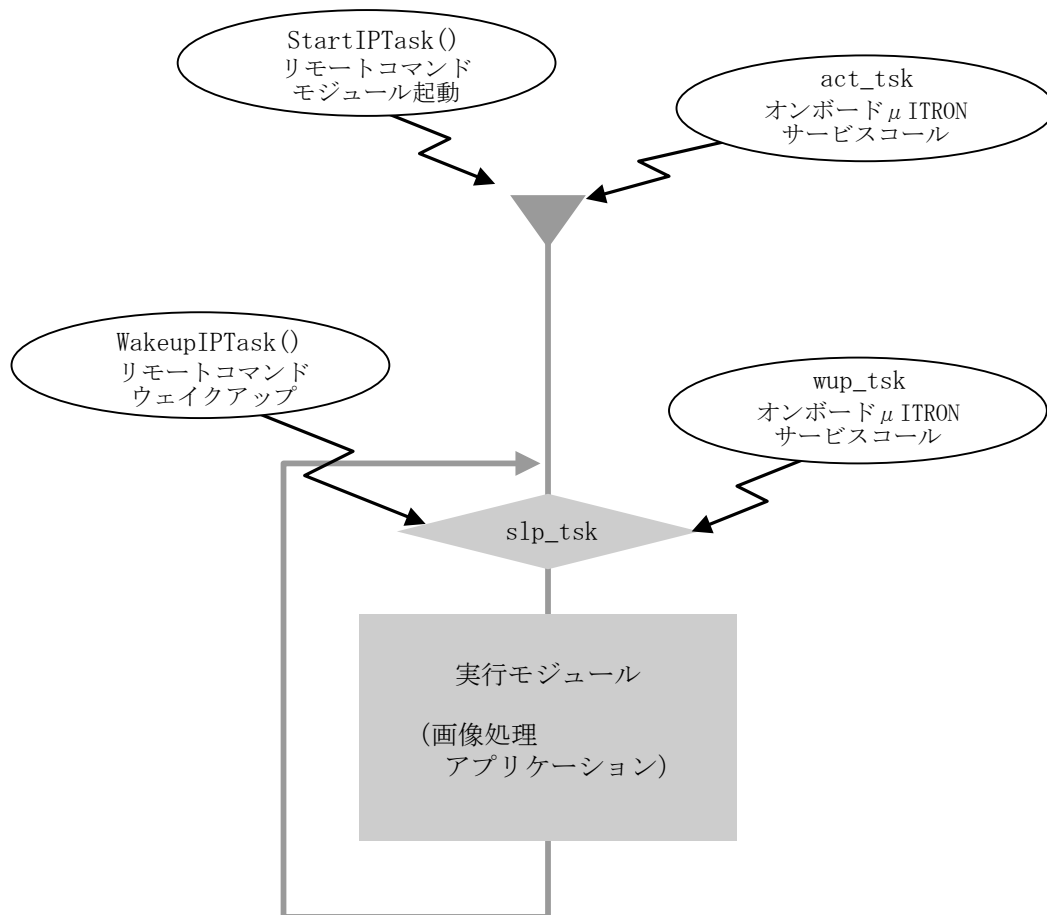
図6-3-1 画像処理タスクモジュールの動作
