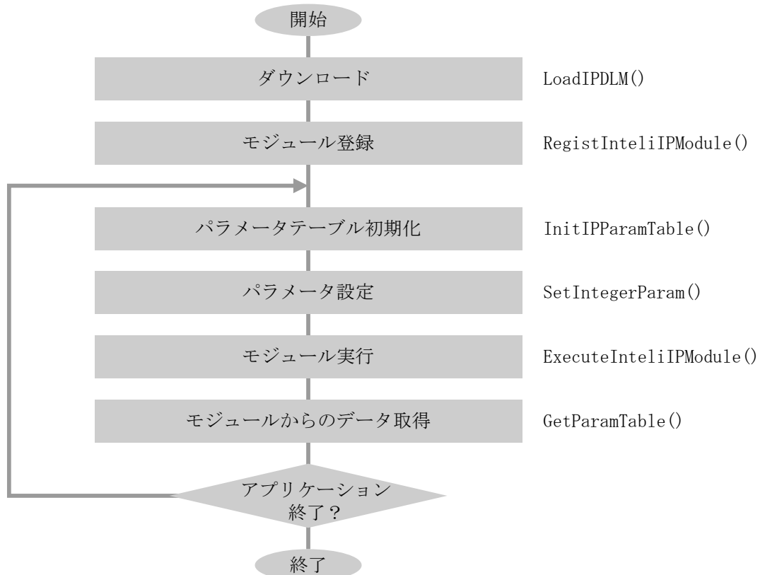
図6-2-2 モジュール実行フロー
