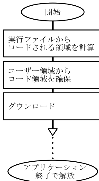
図7-3-1 ロードフロー
