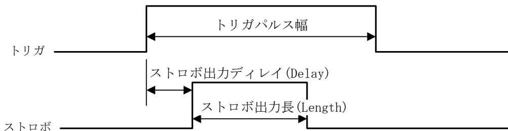
図4-5-11 トリガおよびストロボ出力タイミング
