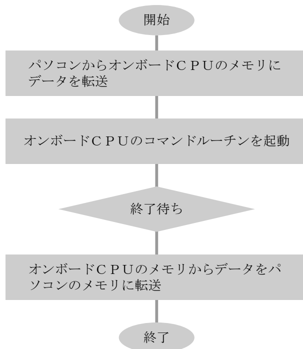
図6-1-1 コマンド実行フロー
