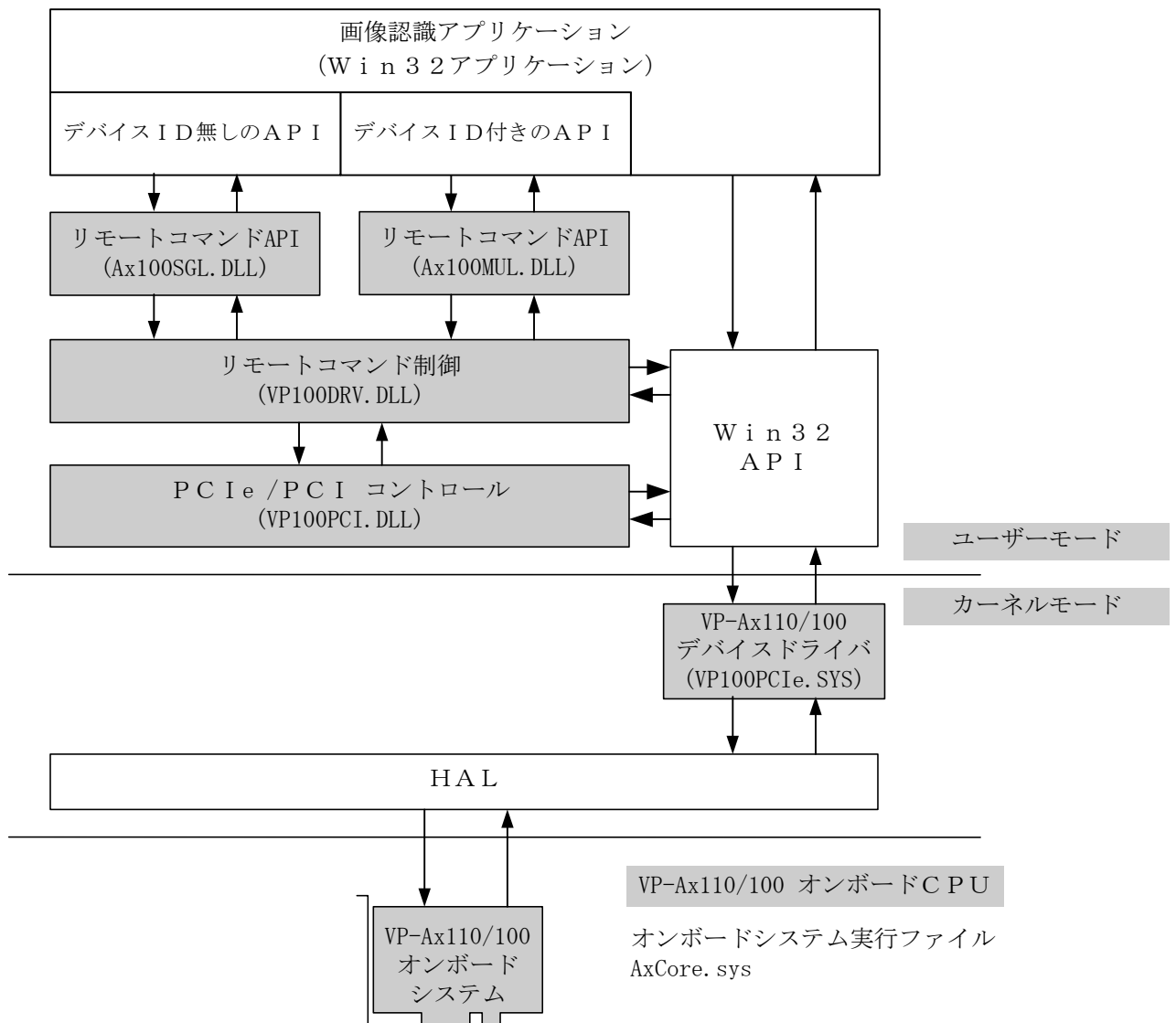
図1-3-1 リモートコマンドの構成
