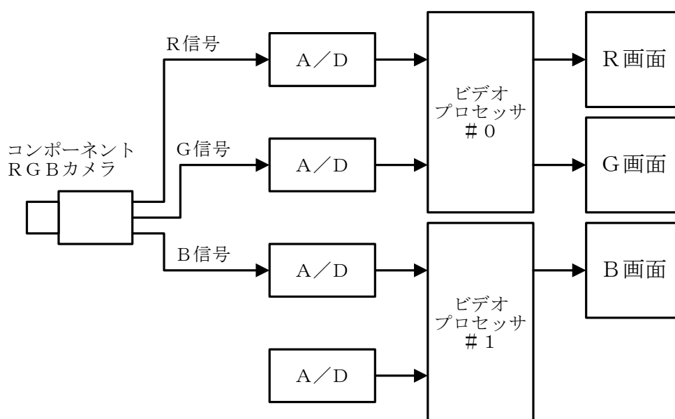
図4-7-2 RGB映像入力部のハード構成
