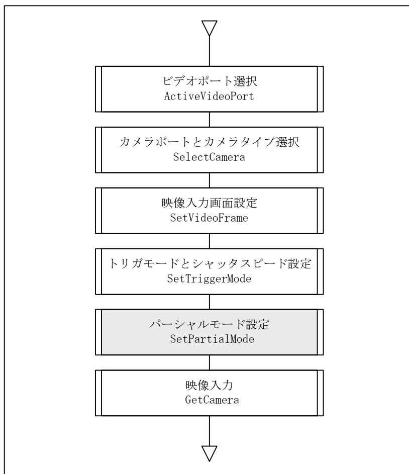
図4-5-13 パーシャル映像入力フロー
