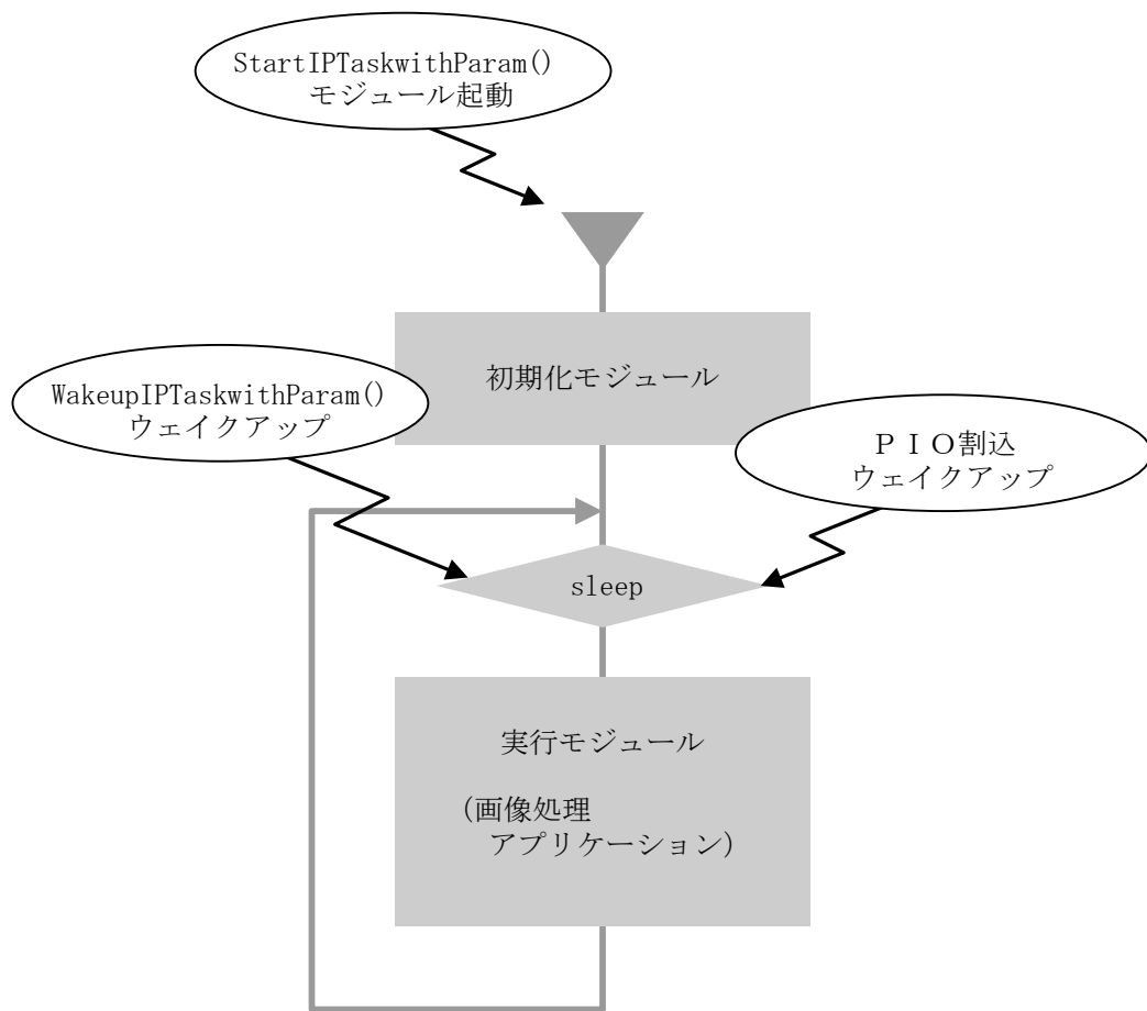
図6-4-4 割込モジュールの動作
