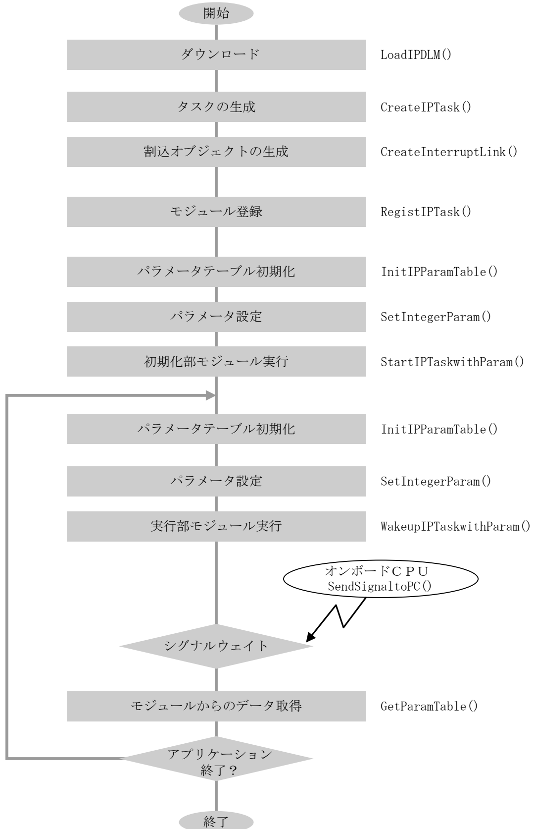
図6-4-5 割込起動モジュール制御フロー
