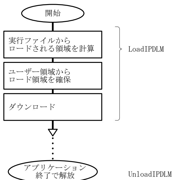
図6-1-2 ロードフロー
