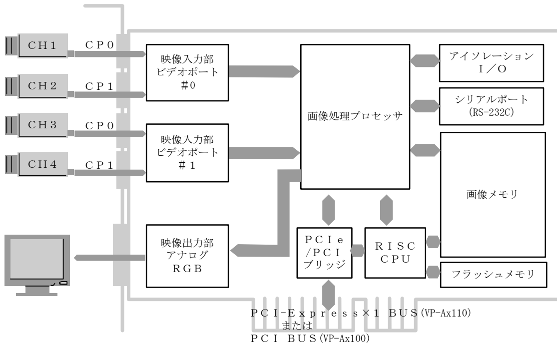
図1-2-1 画像処理ボードVP-Ax110/100
