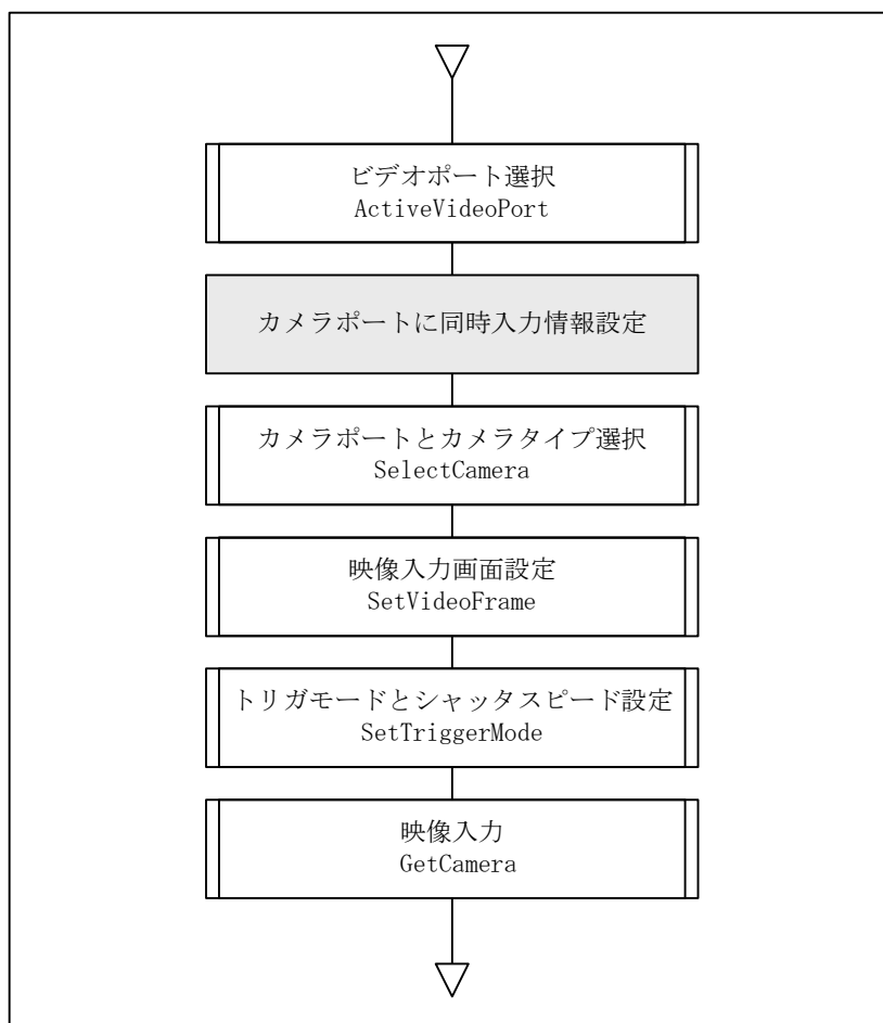
図4-5-9 カメラ同時入力時の映像入力フロー
