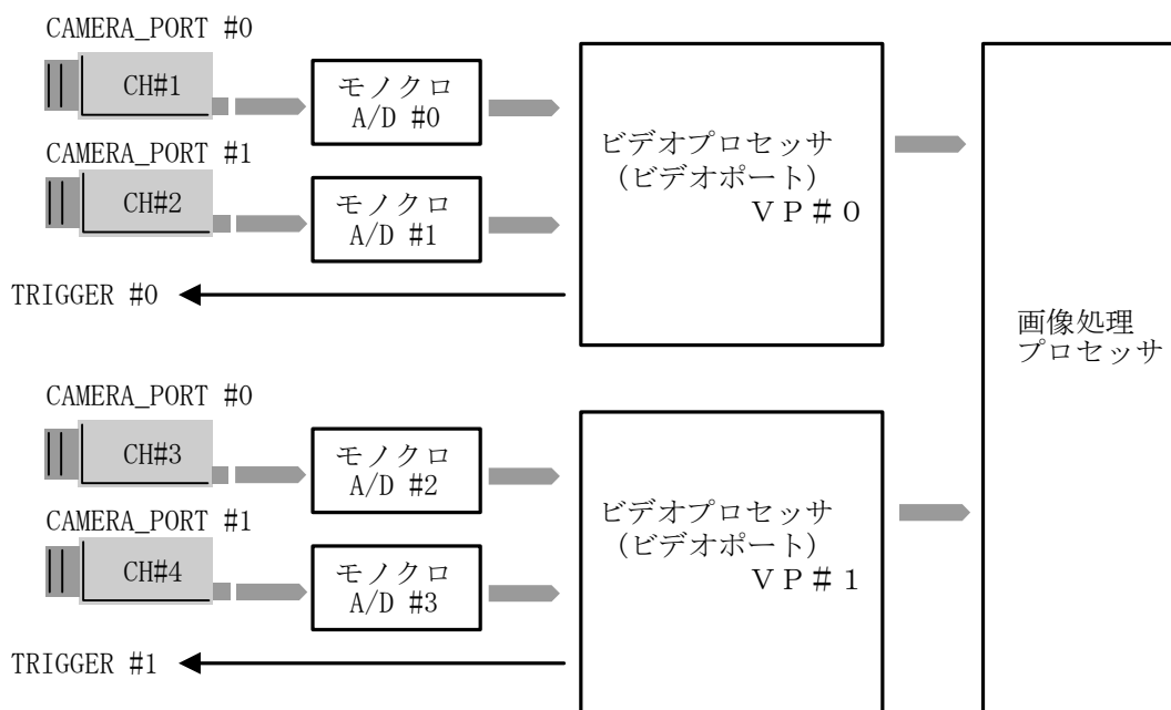
図4-5-1 映像入力ハードウェア構成
