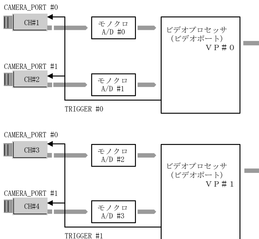
図4-5-8 VP-Ax110/100 チャンネル構成
