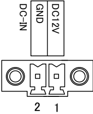
NVP-Ax430ACL/435CL/435FCL
