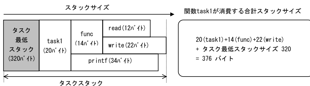
図6-5 タスクのスタック計算方法(SH2A-FPUのとき)
