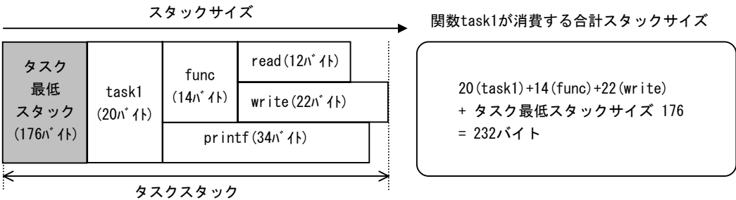
図6-4 タスクのスタック計算方法(SH-2Aのとき)
