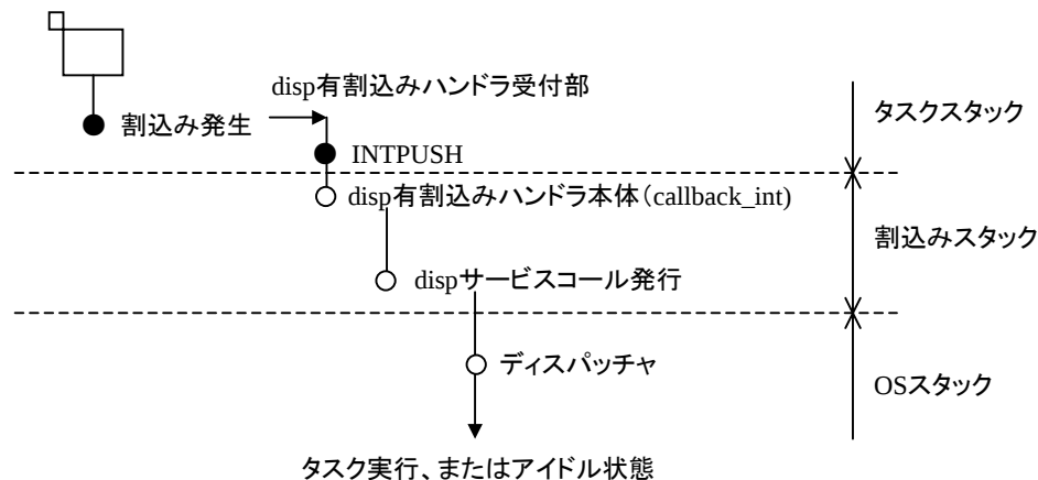
図6-6 disp有割込みハンドラのスタック切り替えタイミング
