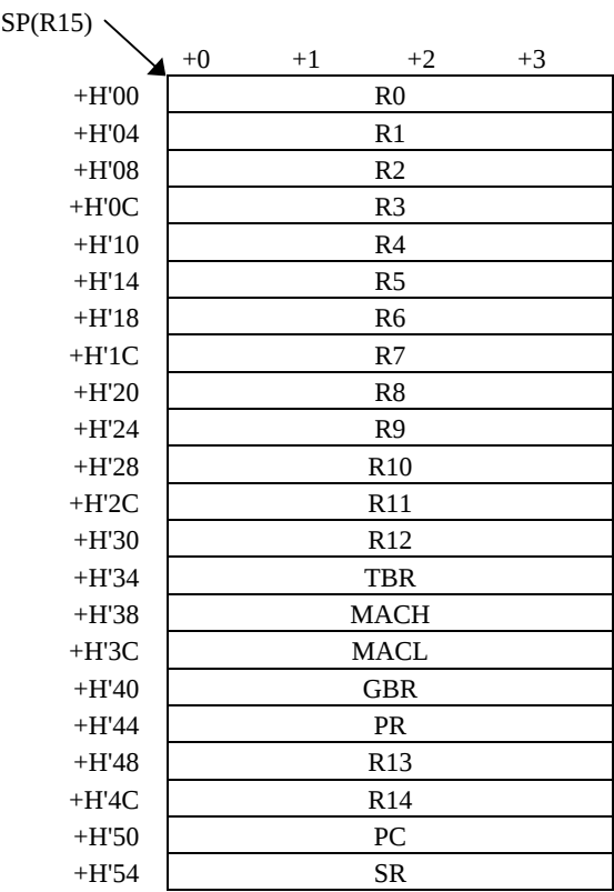
図D-1 SH-2Aのスタック仕様
