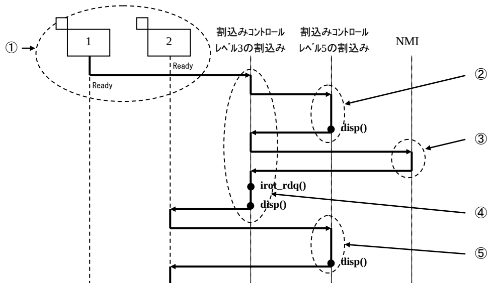
図3-16 多重割込み動作例
