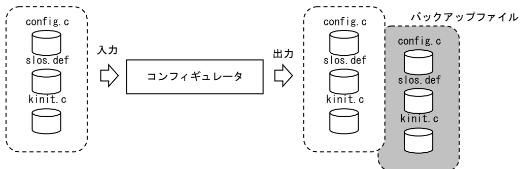
図7-2 Smalight Configuratorの入出力
