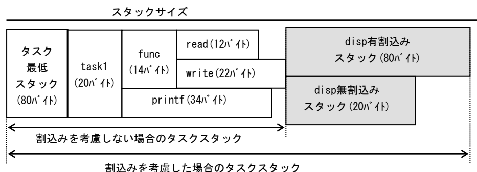
図6-5 タスクスタックとdisp無割込み
