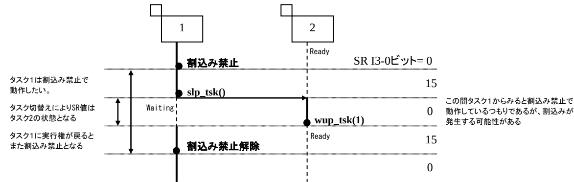
図3-5 割込み禁止状態でのタスク切替え
